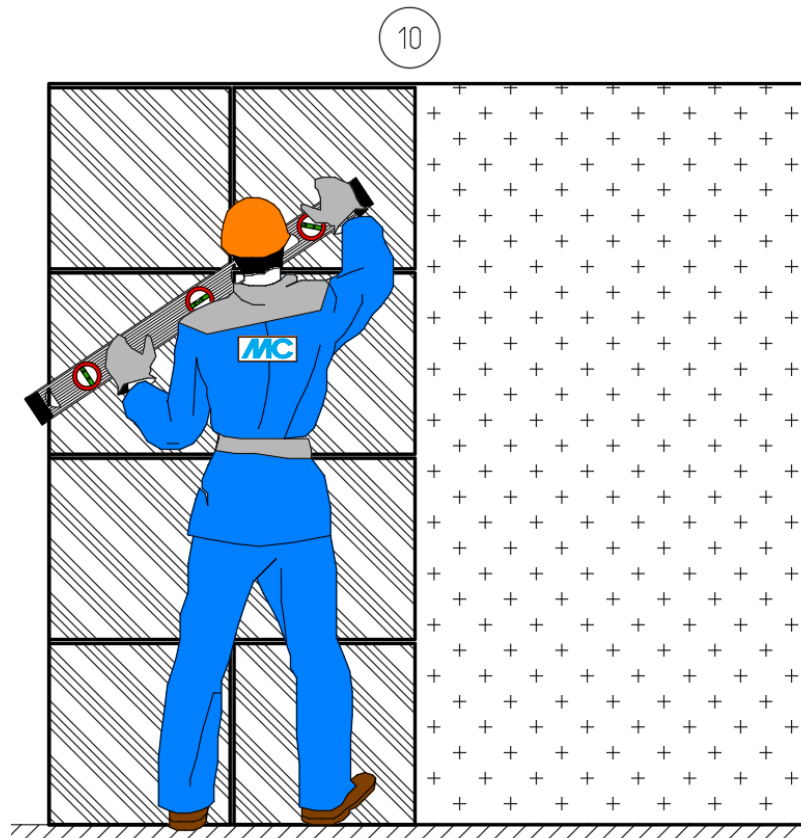
Рис.25. Последовательность работ, где: 1 – проверка ровности основания контрольной рейкой; 2, 3 – приготовление грунтовки; 4 – нанесение грунтовки на цементную штукатурку; 5 – приготовление клеевой смеси; 6, 7 – нанесение клеевой смеси на основание (захватками); 8, 9 – приклеивание керамогранитной плитки на стену (захватками); 10 – проверка облицовки при помощи уровня.
