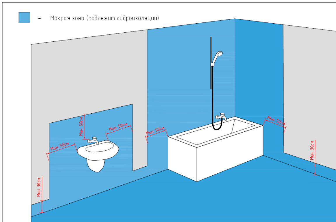
Рис. 23.2 Мокрые зоны внутри влажных помещений, подлежащие гидроизоляции.
